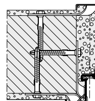
Hjørnekarm og supplerende karm
