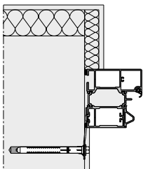
Standardkarm Montering med forankring
