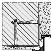
Montering med dyvelforankring
