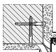
Montering med dyvelforankring
