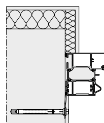
Standardkarm Montering med forankring
