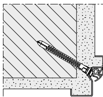
Special-hjørnekarm Gennemskruningsmontering gennem notbunden
