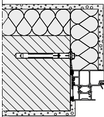
Standardkarm Montering med forankring
