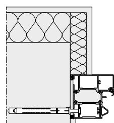
Standardkarm Montering med borehuller
