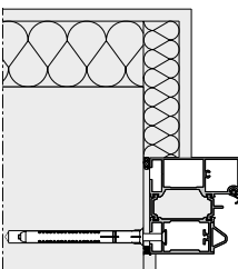
Standardkarm Montering med borehuller
