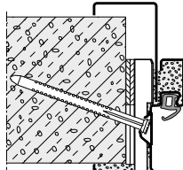
Diagonalfastgørelse med supplerende karm Vario B53 som yderkarm i 2 dele (gasbeton)
