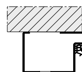
Standardkarm til montering på væggen (profil 006) (kontrolleret på den modsatte side af hængslet)
