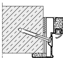
Diagonalfastgørelse (synligt murværk / beton)
