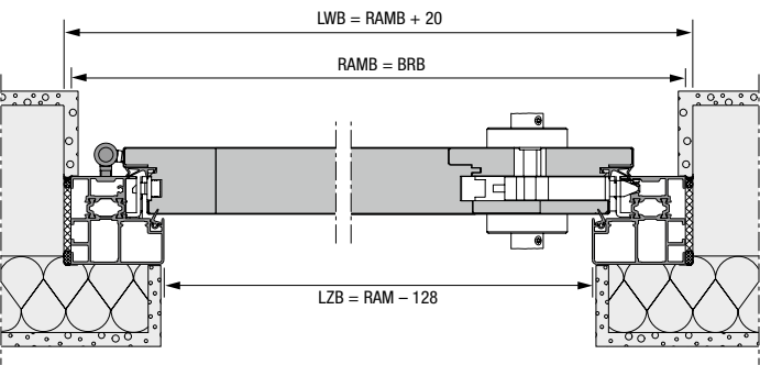
Vandret snit
