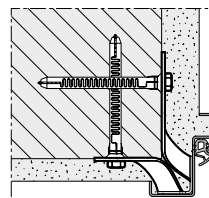
Montering med dyvelforankring
