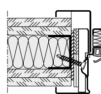
Diagonalfastgørelse (gasbeton)
